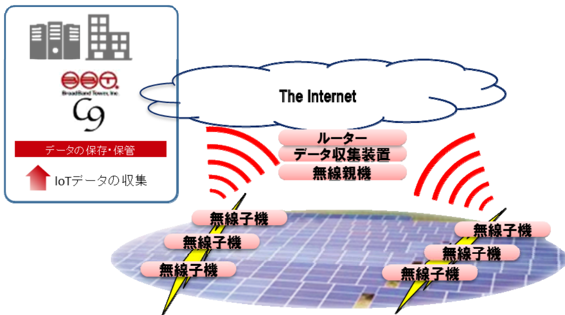
構内無線方式によるストリング監視システムイメージ図
